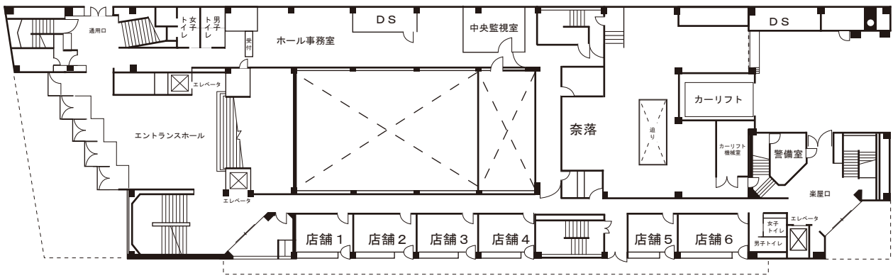
1階平面
